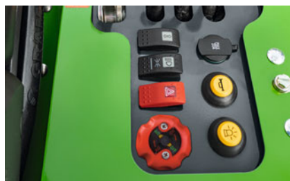
Sezionatore batteria 1
